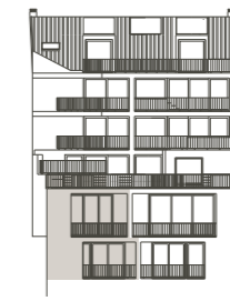
ALÇADO RIO TEJO REAR FACADE FAÇADE ARREËRE
